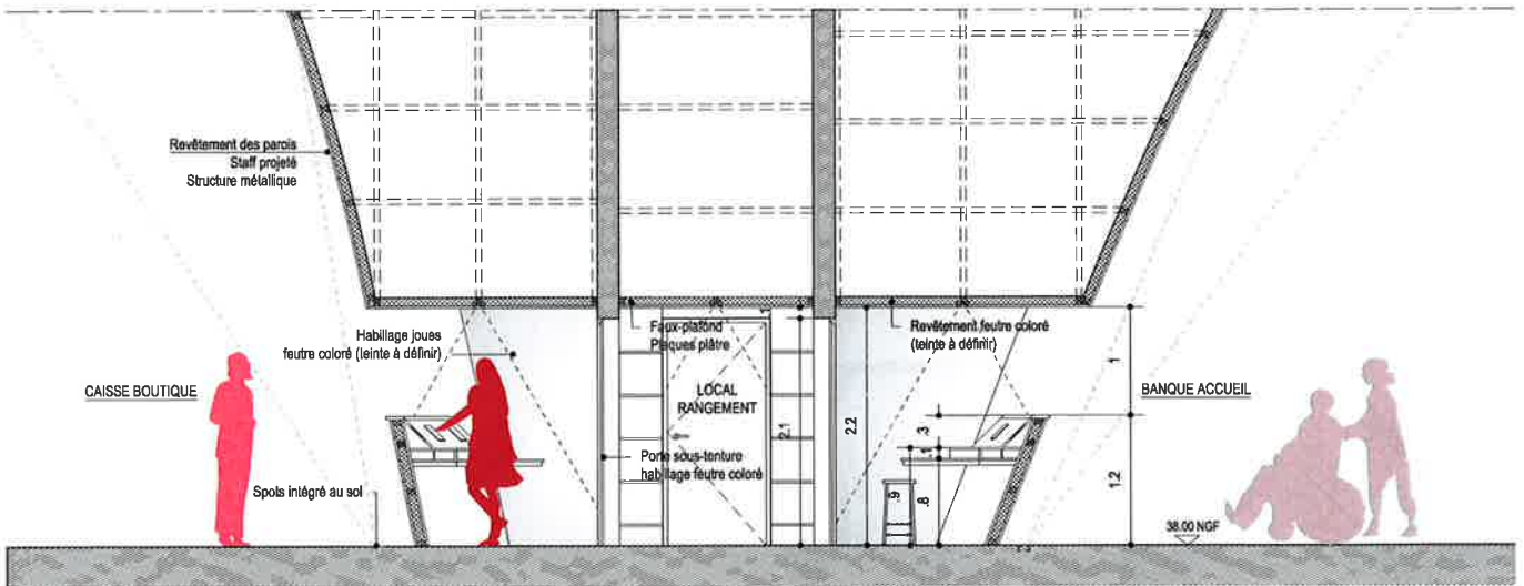
COUPE 1-1'
